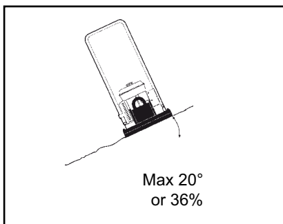
Kaldenurk külgakalatel
